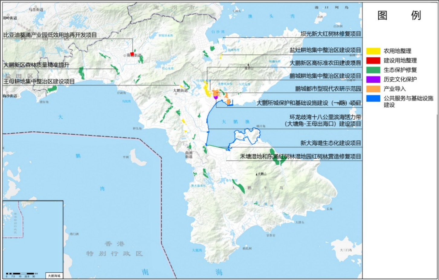
深圳市大鹏新区全域土地综合整治项目分布图
